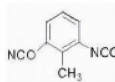
2,6-TDI
